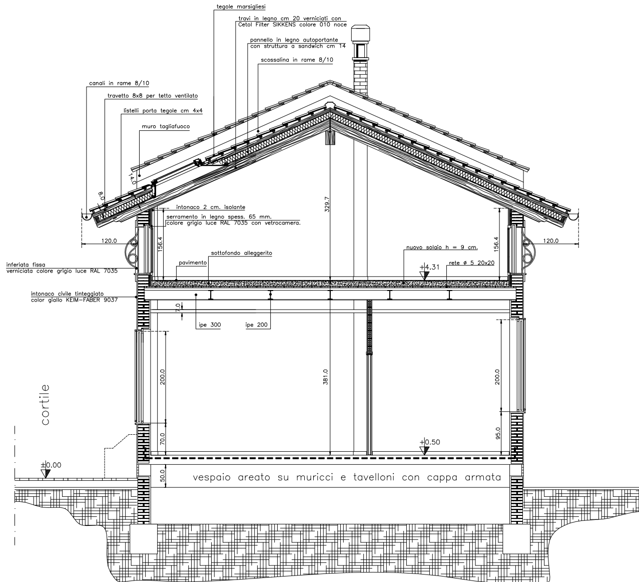
SEZIONE X-X
